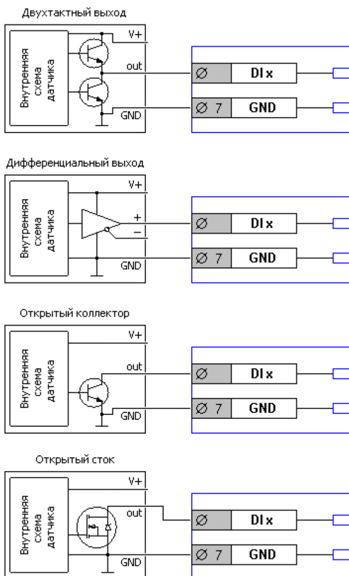
Рис. 35 -Схемы подключения датчиков с различными типами выходов
